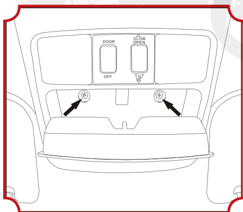
شکل ۷-۵۷ باز کردن چراغ بالا جلو
