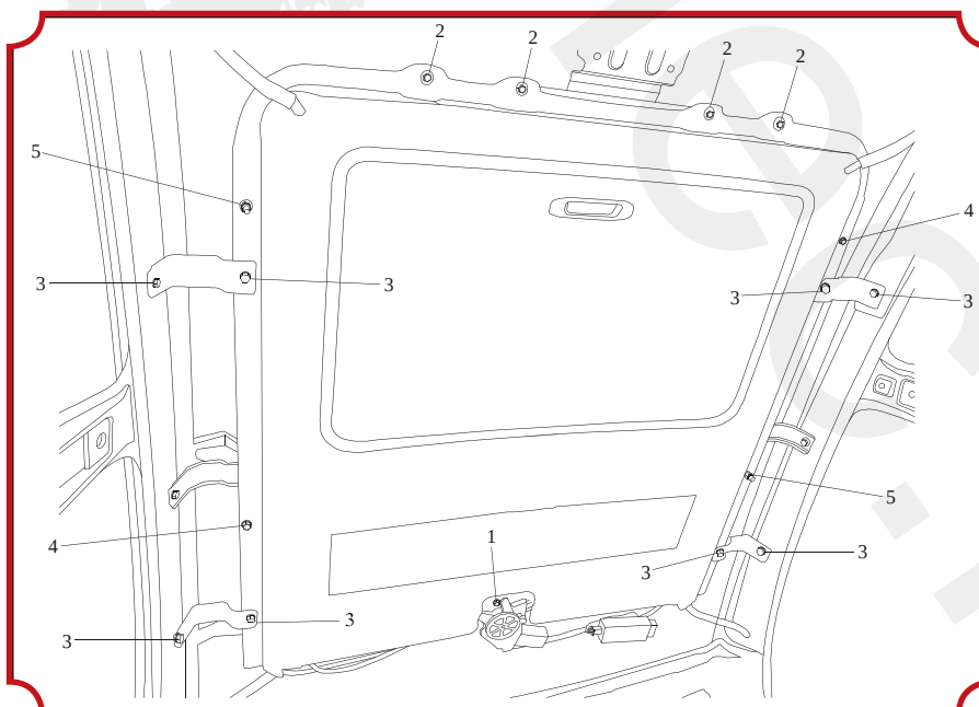
شکل ۵۹- باز کردن مجموعه شیبداغ
