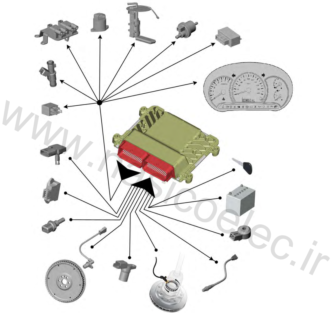
سنسورها و عملگرهای مرتبط با ECU
