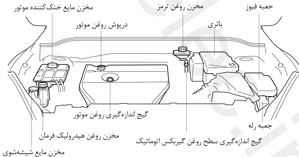
موتور 2.0 MZR
