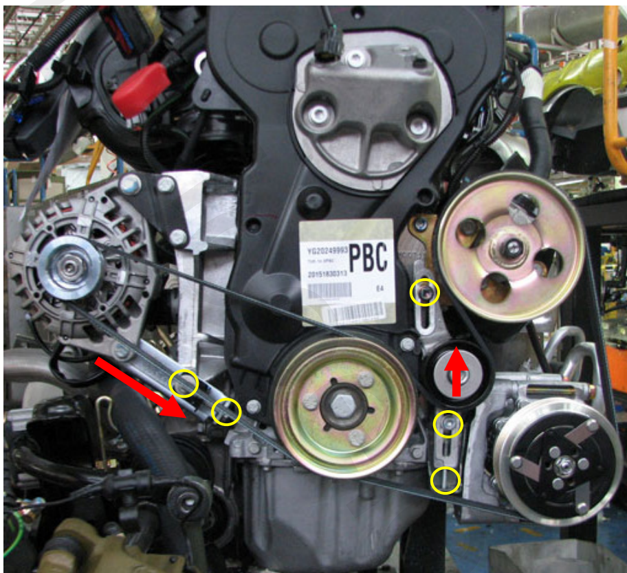
موتور ۵TU در خودروهایی پژو ۴۰۵، پارس و سمند
