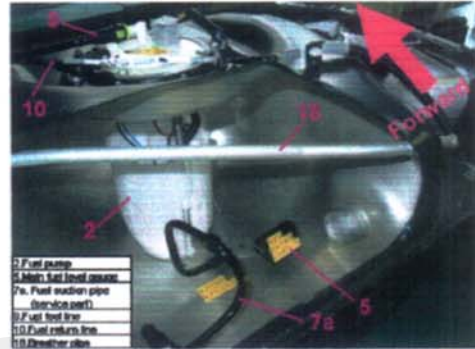
۱۵۸۰۱۰۰۹ گیج داخل باک بنزین با پمپ و فیلتر
