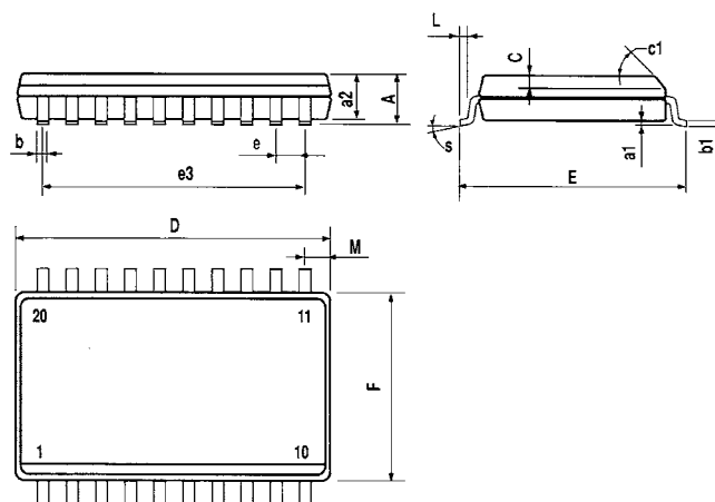
SO 20 (300 mil JEDEC-STD)
