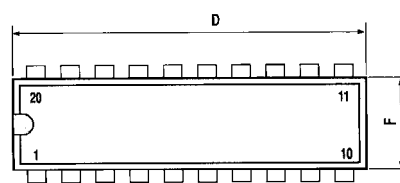
DIL 20 (300 mil JEDEC-STD)
