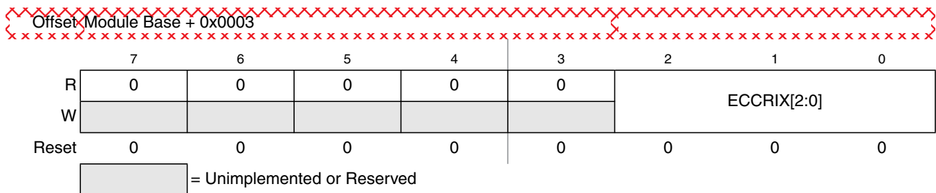
Figure 29-8. FECCR Index Register (FECCRIX)
